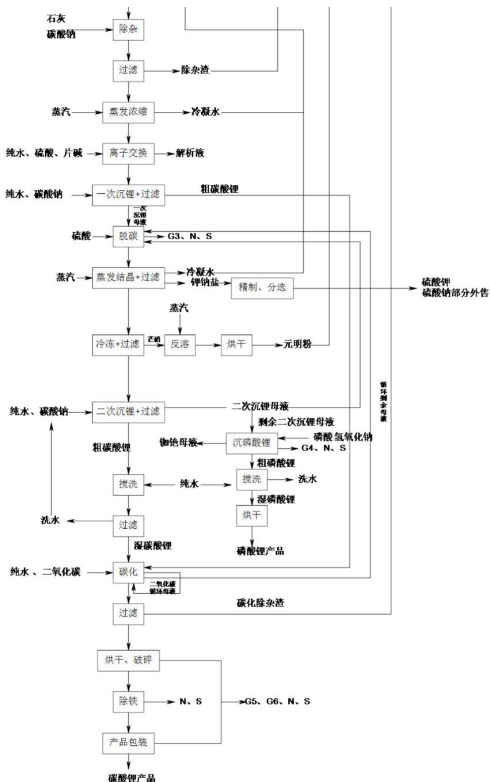
图 1 碳酸锂生产工艺流程及产污节点图
